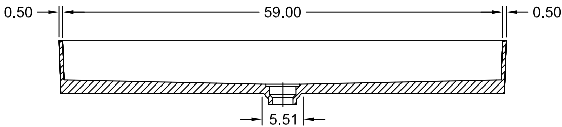
SECTION A-A
